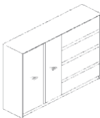
[ BA-C2T4W1612L ] W: 161,5 / D: 40 / H: 120
