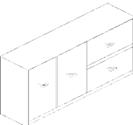
[ BA-C2T2W1608R ] W: 161,5 / D: 40 / H: 80
